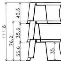
180°反転積層時
