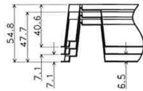
同方向積層時 UNDER STACKS DEPTH 6.5
